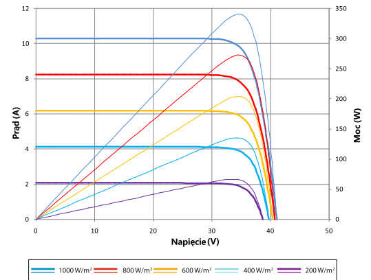
Krzywa prądowo-napięciowa i mocowo-napięciowa (340S)
